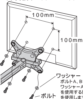
ボルトA〔M4×8〕 ボルトB〔M4×12〕 ボルトC〔M5×8〕 ボルトD〔M5×12〕
